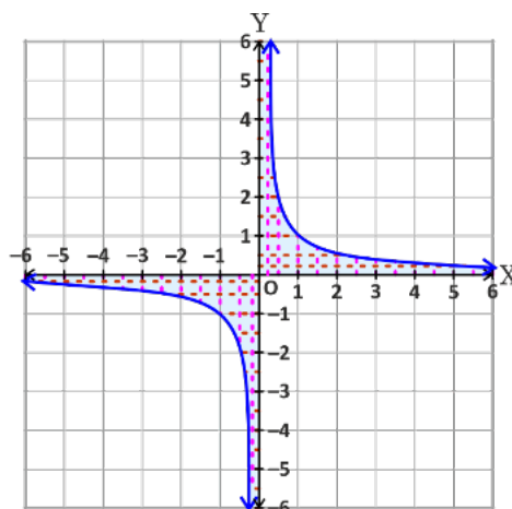
Domain : x \in (-\infty, 0) \cup (0, \infty)
